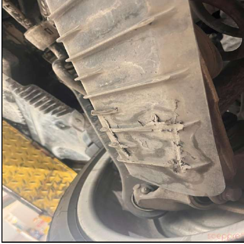
SAĞ ARKA TORSYONUN PLASTİK MUHAFAZASINDA SÜRTME VAR
